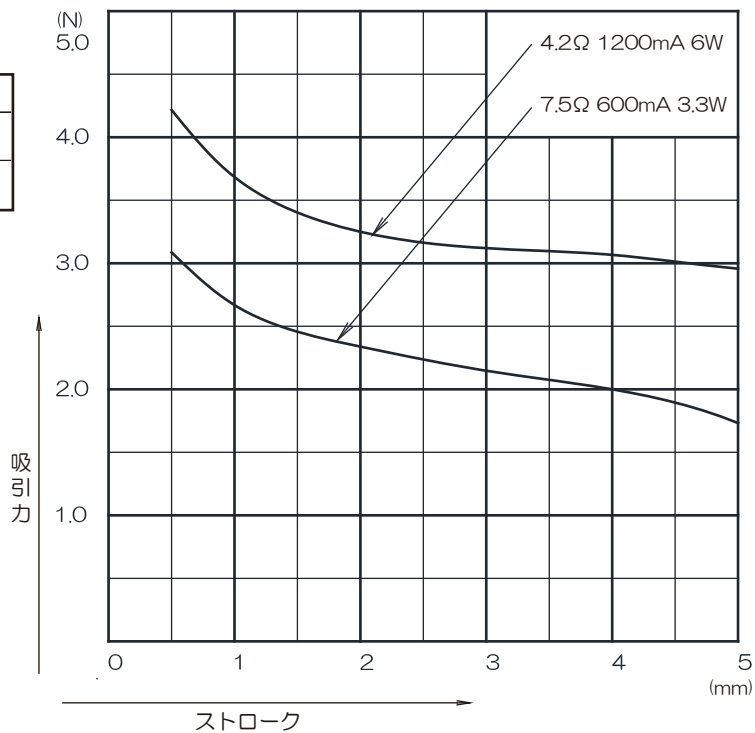
吸引力 - ストローク特性 (DC5V 温度上昇前 周囲温度20°C)
